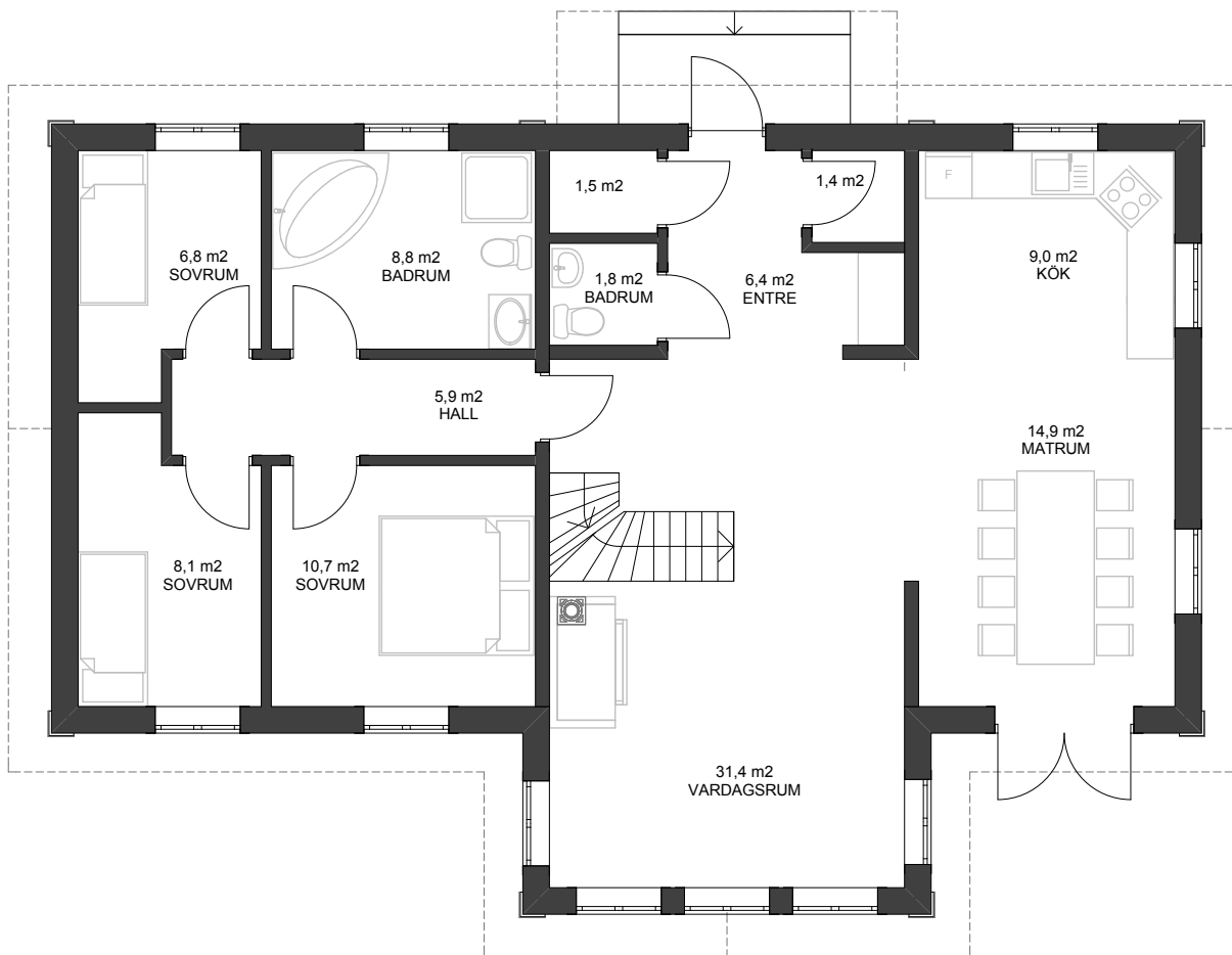
PLAN 1 1:100
